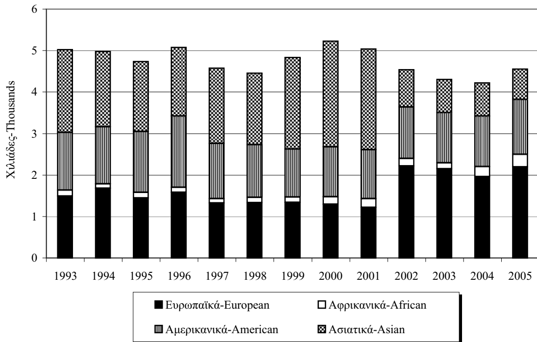
ΔΙΑΓΡΑΜΜΑ 5. ΠΛΟΙΑ ΠΟΥ ΠΡΟΣΕΓΓΙΣΑΝ ΣΕ ΚΥΠΡΙΑΚΑ ΛΙΜΑΝΙΑ ΚΑΤΑ ΕΘΝΙΚΟΤΗΤΑ 1993-2005 FIGURE 5. VESSELS CALLED AT CYPRUS PORTS BY NATIONALITY 1993-2005
